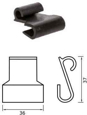
GANCIO SPONDA S LARGO
