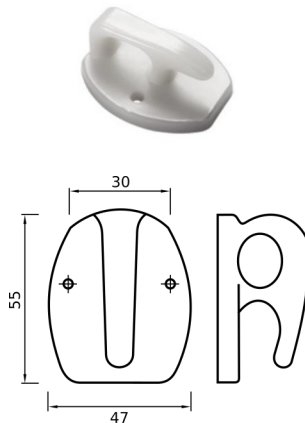
GANCIO COBRA GRANDE
