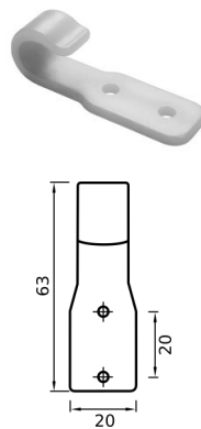
GANCIO ZIG-ZAG APERTO
