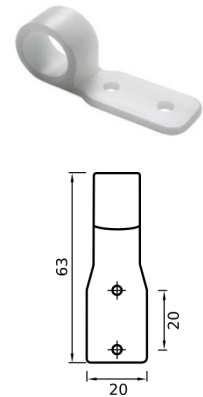
GANCIO ZIG-ZAG CHIUSO
