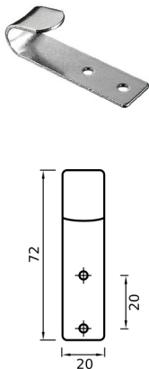
GANCIO SPONDA
