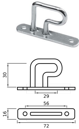
CAVALLOTTO 2 FORI PIPA
