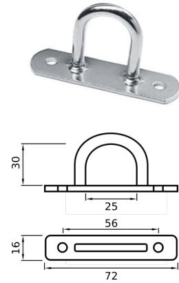
CAVALLOTTO 2 FORI TONDO
