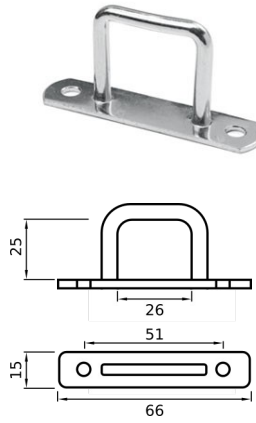
CAVALLOTTO 2 FORI
