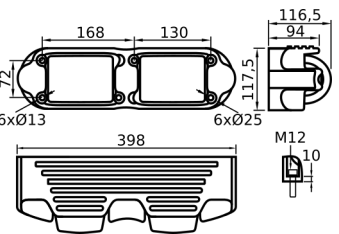
S-ROLL H2 ORIZZONTALE
