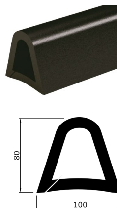
TAMPONE PARACOLPI TIPO ALTO
