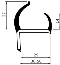
PROFILO IN PVC COESTRUSO
