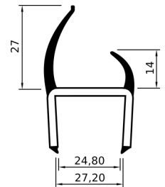
PROFILO IN PVC COESTRUSO
